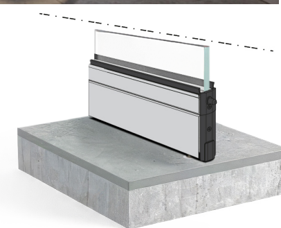
Sistema SK200 (pormenor).
